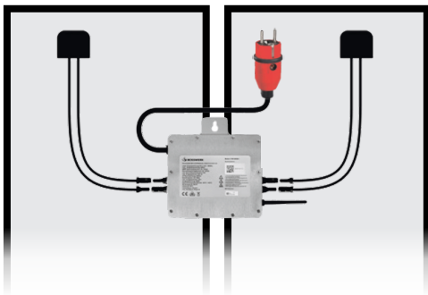
Schema einer Solaranlage mit Wechselrichter
