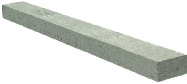
Stahlbetonsturz 1250 x 115 x 71 mm ca. 24 kg - ca. 10 € Baumarkt (auch in 1500 Länge ca 28,5 kg))
